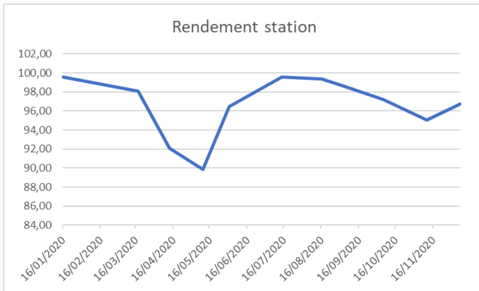
Rendement Station en DBO (en %)
