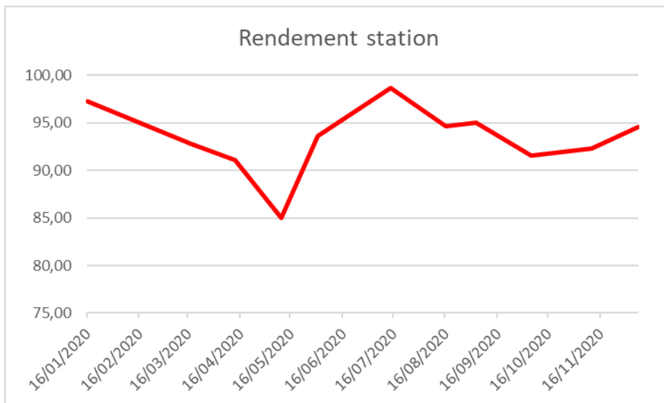
Rendement Station en DCO (en %)
