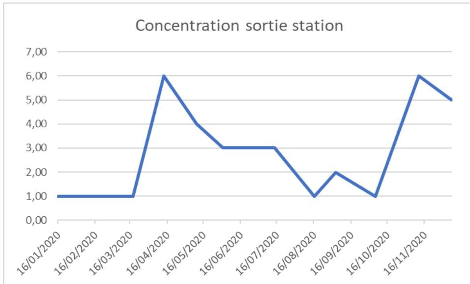
Concentration en sortie de Station en DBO (mg/l)
