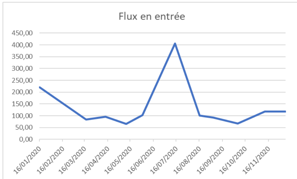
Flux en entrée de Station en DBO (kg/j)
